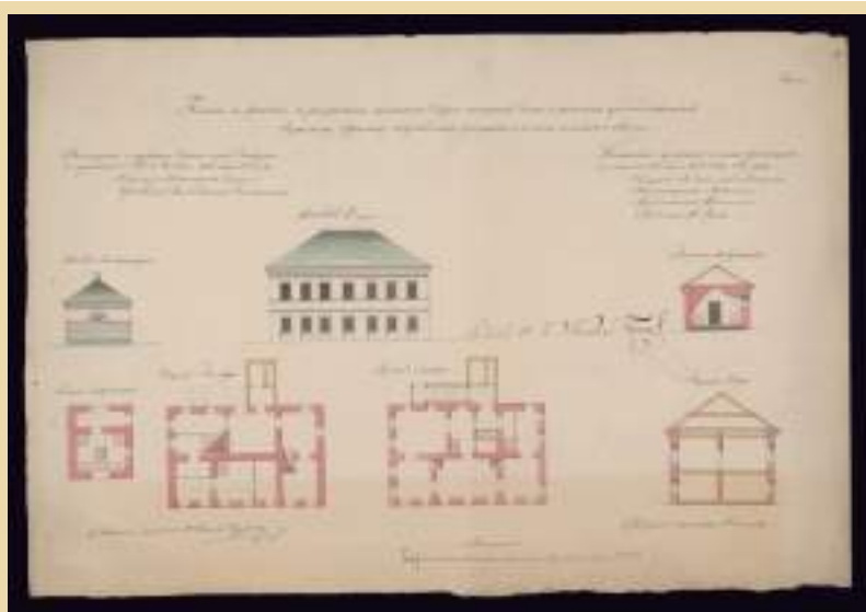
Планы и фасады с разрезами каменного двухэтажного дома и флигеля, принадлежащих Пермскому приказу Общественного призрения, в котором помещается аптека. 1838 г. // РГИА. Ф. 1488. Оп. 3. Д. 256. Л. 2.
