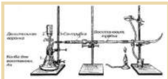
Прибор Марша для определения мышьяка
