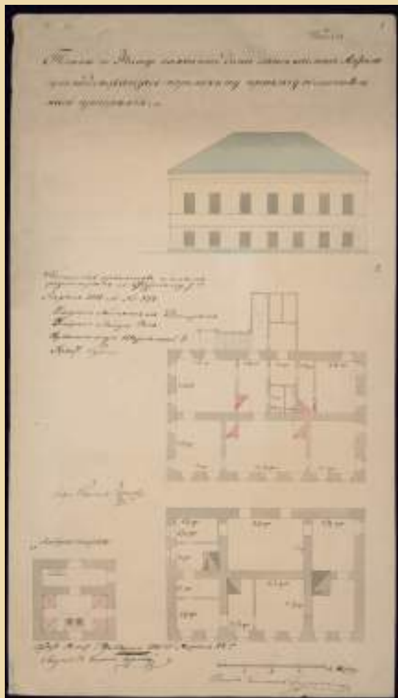
Планы и фасад каменного дома, занимаемого Аптекой, принадлежащего пермскому Приказу Общественного призрения. 1841 г. // РГИА. Ф. 1488. Оп. 3. Д. 256. Л. 2.
