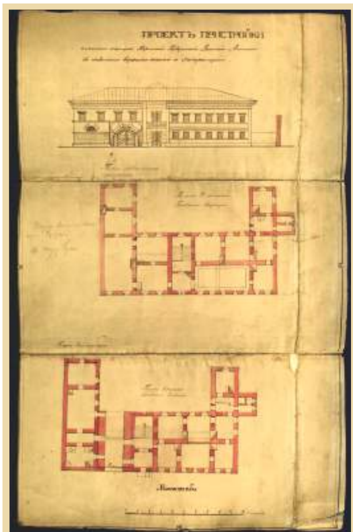
Проект пристройки головного корпуса Пермской губернской земской аптеки для соединения верхнего этажа с лабораторией // ГАПК. Ф. 279. Оп. 5. Д. 452. Л. 1.
