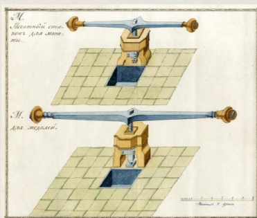
Оборудование, использовавшееся на Санкт-Петербургском монетном дворе. Из альбома А. А. Нартова «Описание монетного производства со изображением плавильных печей и действующих машин». 1779 г. Российская государственная библиотека
